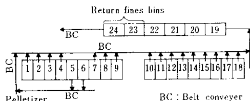
Fig. 4 Raw material bins
