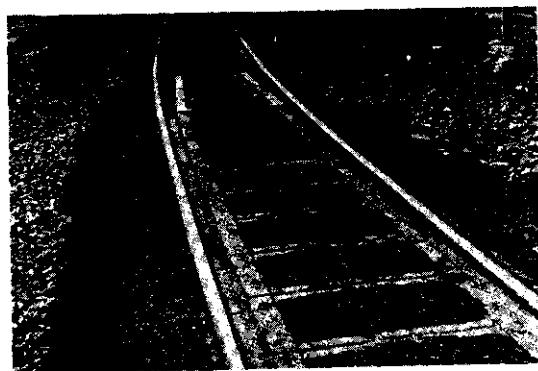
写真11 合成タール混合鉱滓バラス踏切 (組立式)
