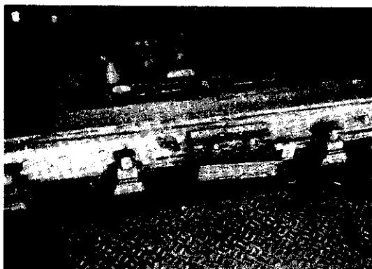
写真 15 クレーンレール74kg締結 (3枚の楔形継目板, 継目部)
